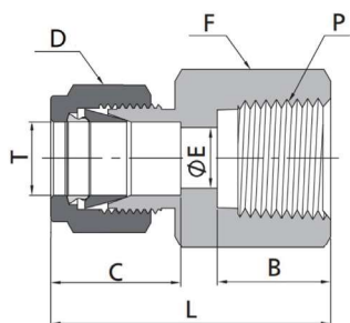
公制管-RT内螺纹/Metric Tube to RT Thread
